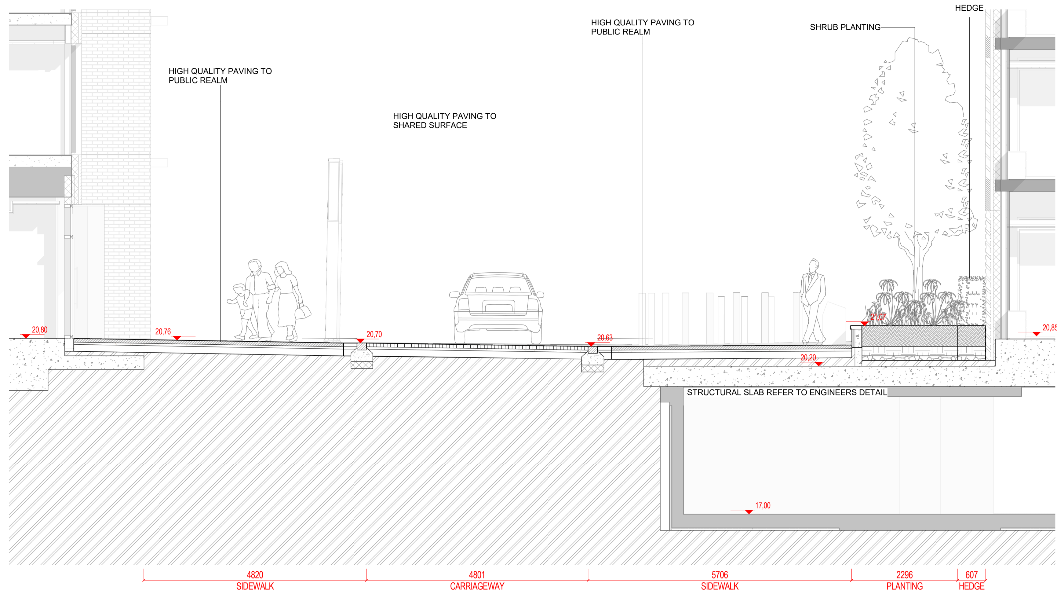
4 SECTION 22 1:50 @A1
