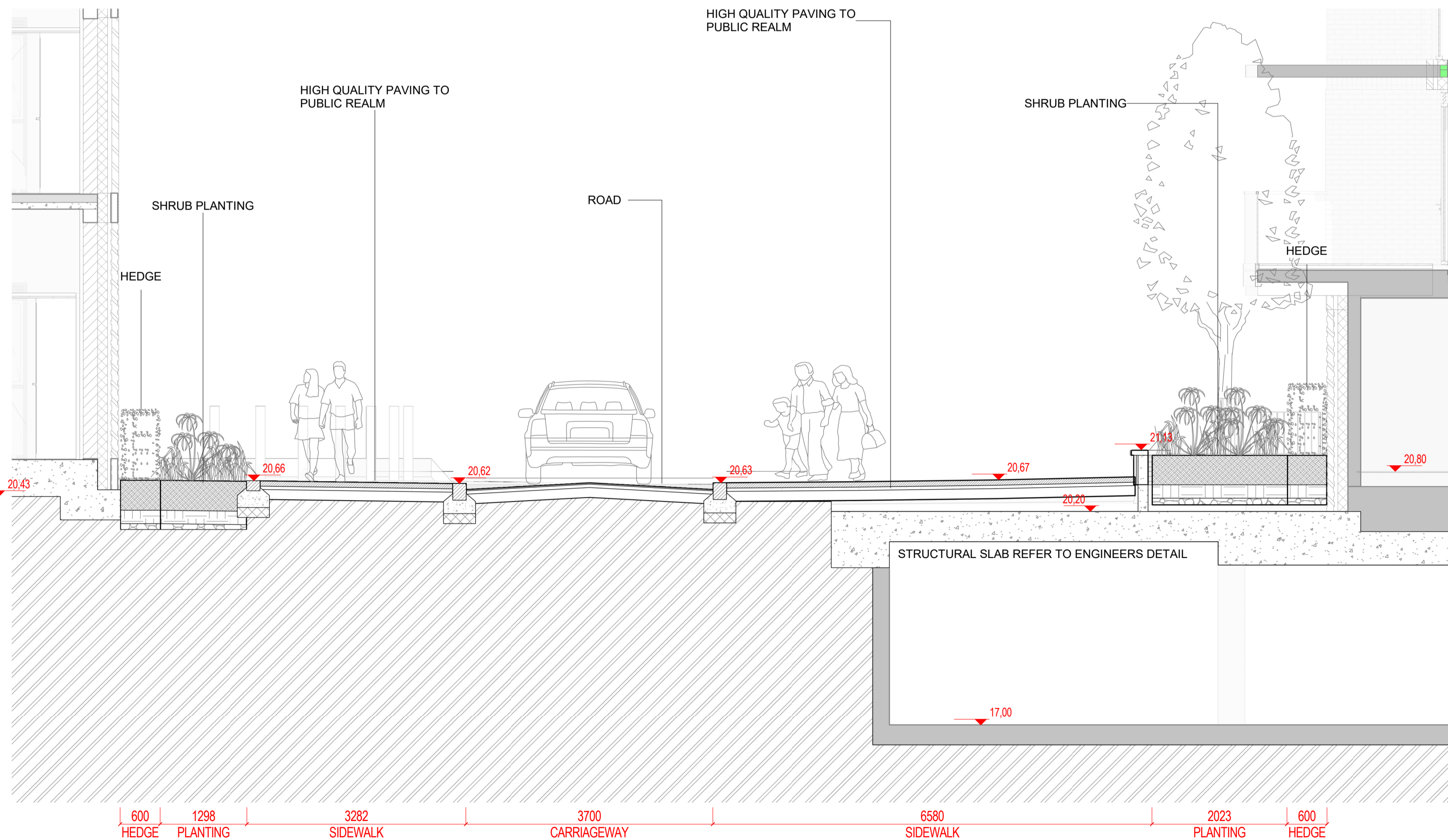
1 SECTION 23 1:50 @A1
